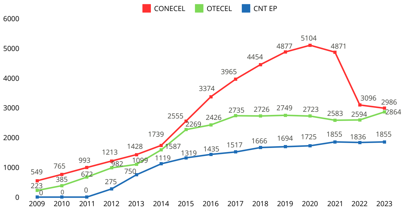
FIGURA 12.EVOLUCIÓN RBS TECNOLOGÍA 3G INSTALADAS POR PRESTADOR
