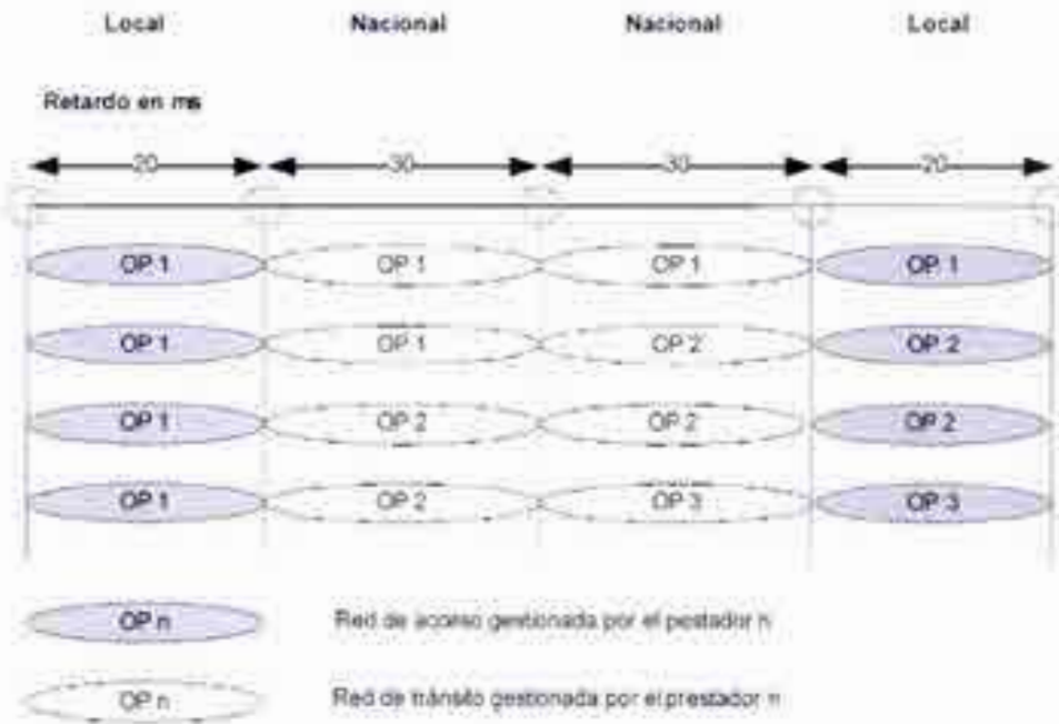
Figura 7 - Distribución de retardos de transmisión en el circuito nacional
