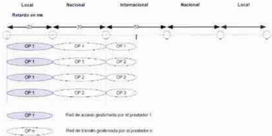
Figura 6 - Distribución de retardos de transmisión en el circuito internacional
