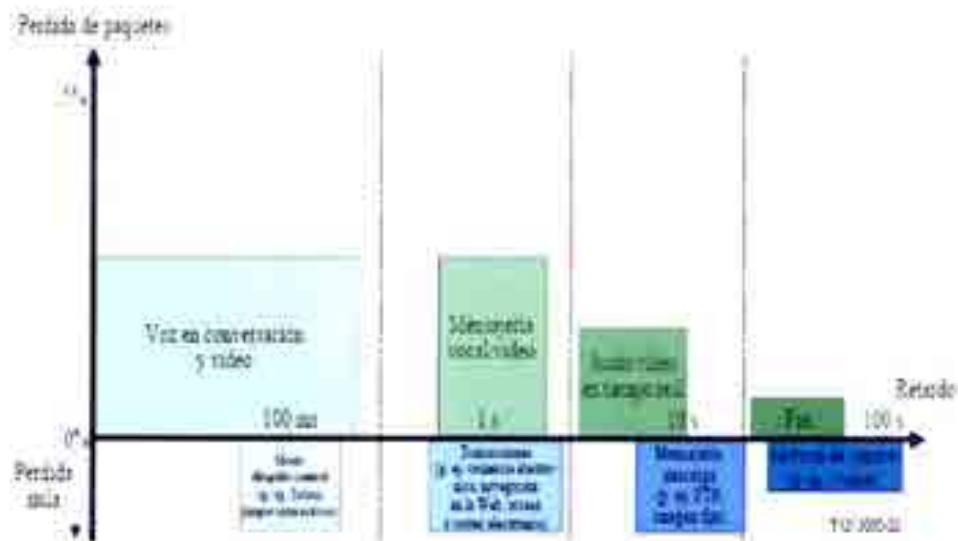
Figura 1- Correspondencia entre requisitos de QoS de usuario y servicios
